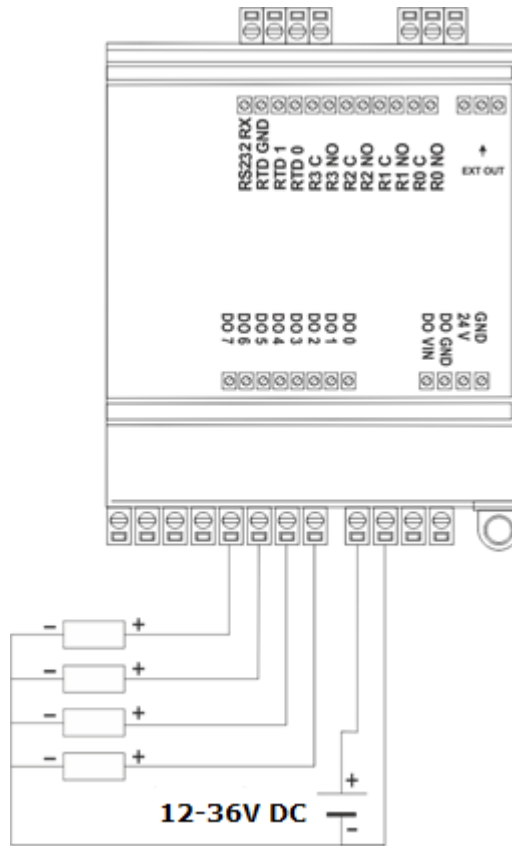
Şekil 9 Dijital Çıkış Bağlantı Şeması
