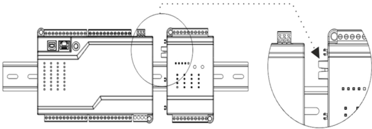
Şekil 2 Genişleme Modülü Montajı
